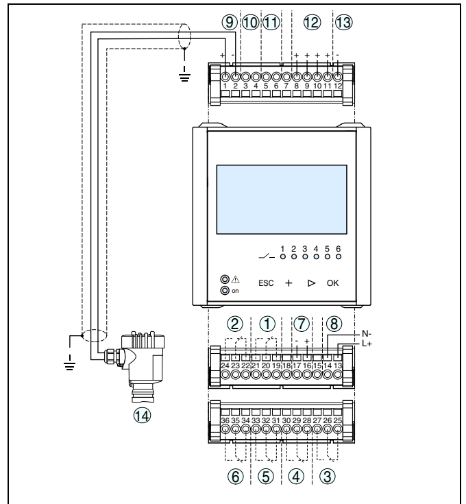
Рис. 14: Схема подключения с двухпроводным датчиком
