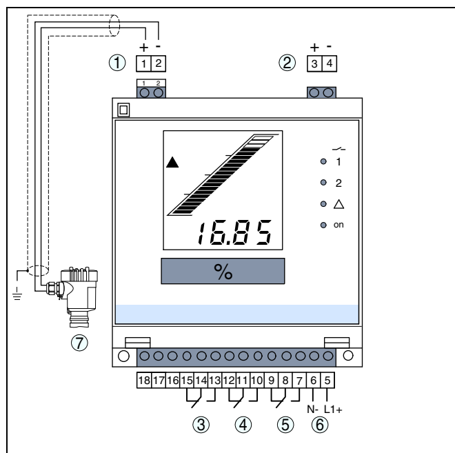
Рис. 12: Схема подключения с двухпроводным датчиком
