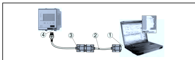
Рис. 24: Подключение ПК через RS232
