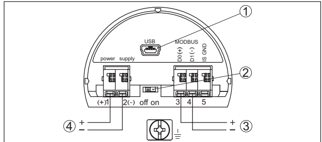
Рис. 6: Отсек подключения
