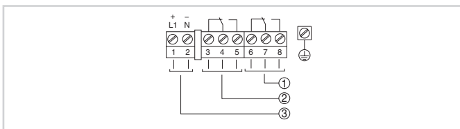
Схема подключения
