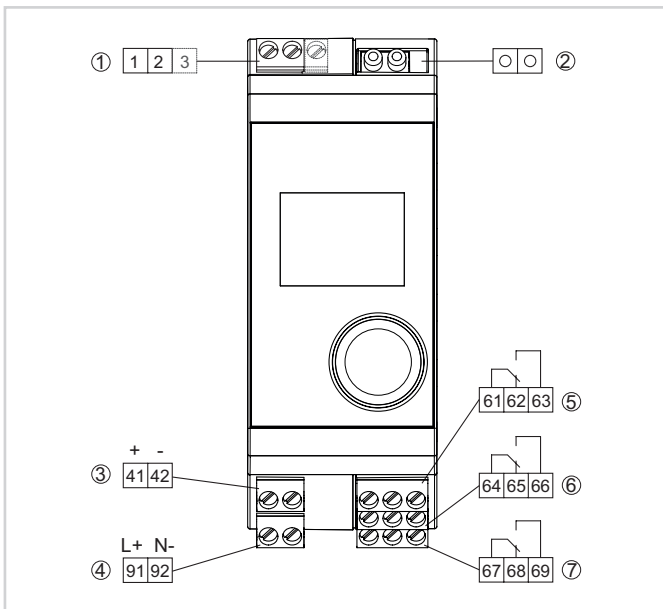
Схема подключения VEGAMET 141
