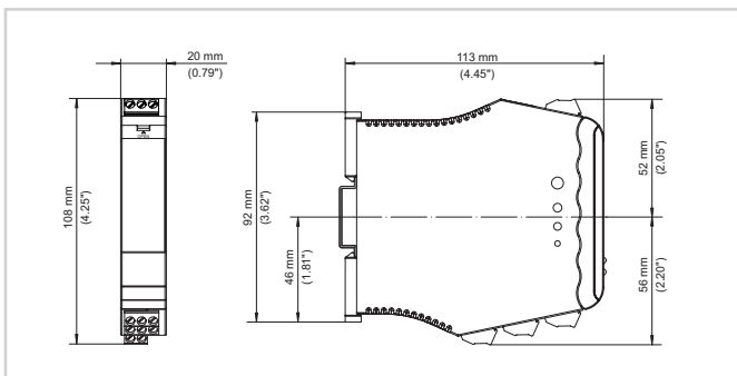
Размеры VEGATOR 142
