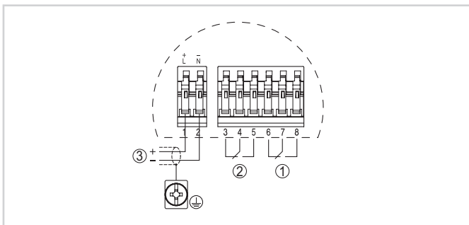
Схема подключения
