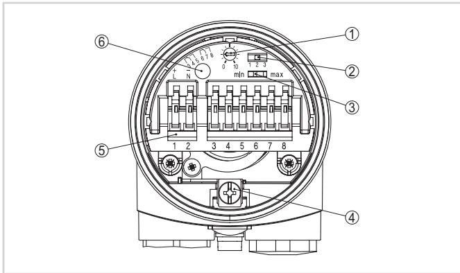
Блок электроники с релейным выходом
