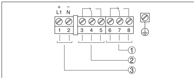
Рис. 7: Схема подключения
