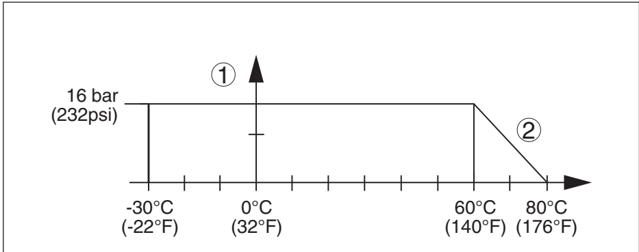
Рис. 25: Давление процесса - температура процесса - VEGACAP 35 с присоединением из алюминия
