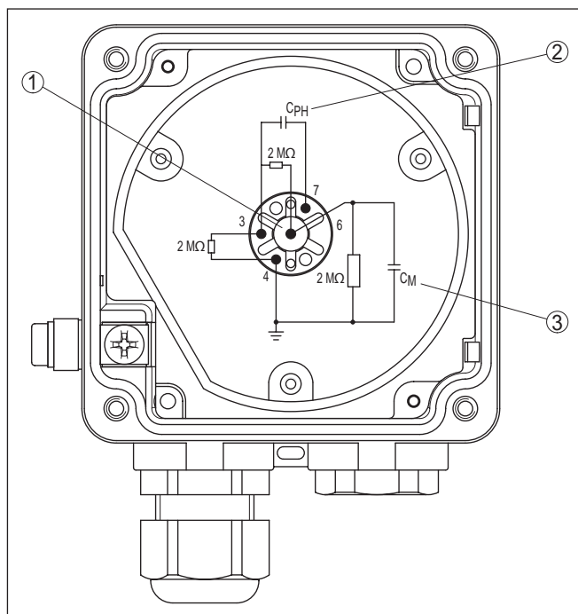
Рис. 23: Проверка сопротивления внутри измерительного зонда
