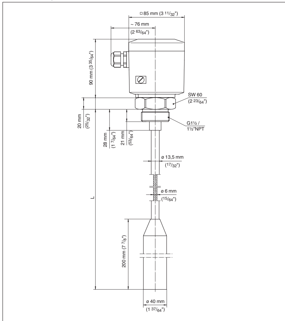
Рис. 28: VEGACAP 35, тросовое исполнение \phi 6 \text{ мм} , резьба G1\frac{1}{2} (ISO 228 T1)
