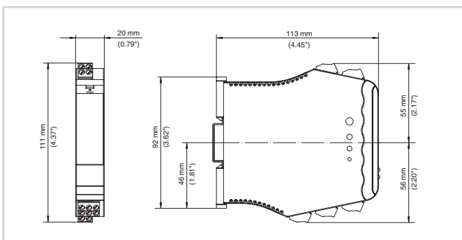
Размеры VEGATOR 112
